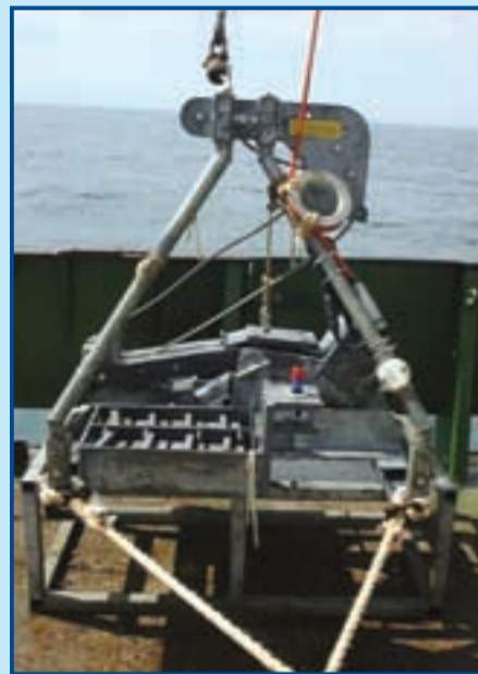
Hamon Grab
